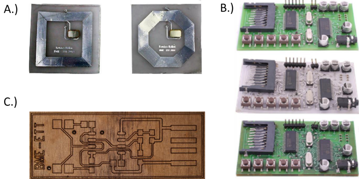
2.ábra. A: RFID címkék, B: MP3-as lejátszók FR4, PLA és GPTe-DETDA hodoszókön, C: Additív Ag+Cu rétegfelvitel lézeres rajzolattal.
